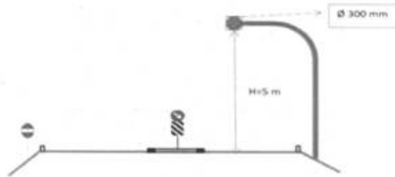
Şekil 2 L Şeklinde Profil Üzerinde Kırmızı Flaşör Sistemi
